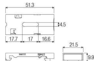
取付けブラケット
