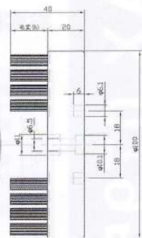
Ø100タイプ図
